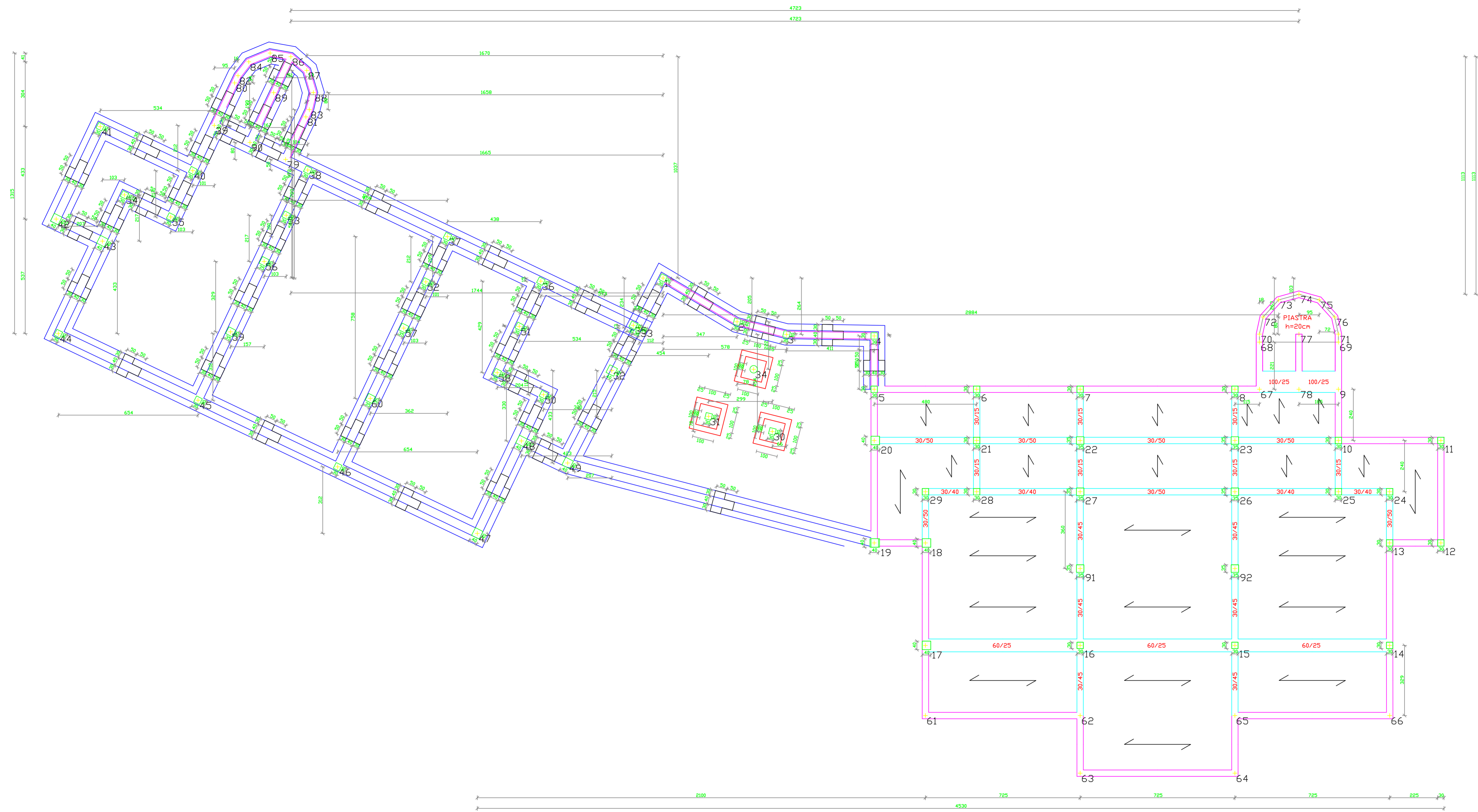
PIANTA IMPALCATO QUOTA m: 3.40
