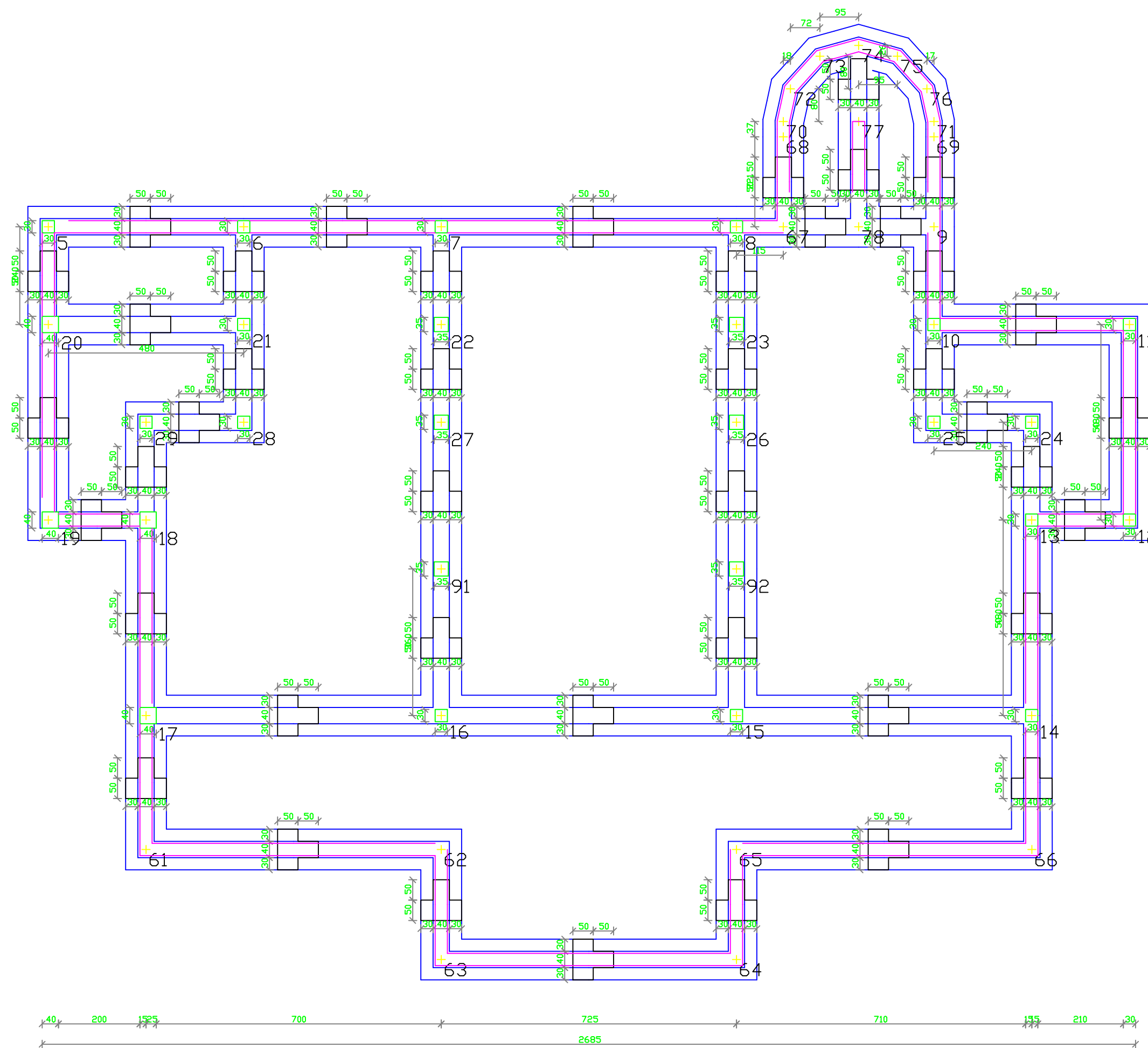
PIANTA IMPALCATO QUOTA m: 0.00
